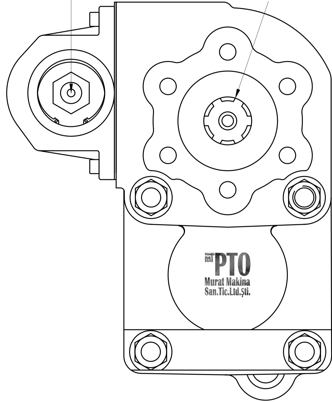
6 Kamalı Frezeli Mil 6x21x25 21 UNI 222
