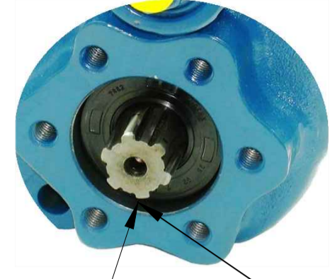
6 Kamalı Frezeli Mil 6x21x25 21 UNI 222
